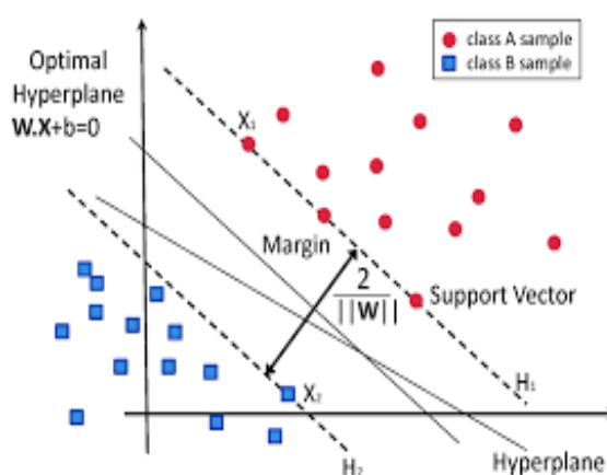
Hình 1.1. Mô hình thuật toán SVM ( https://www.researchgate.net/figure/Classification-of-data-by-support-vector-machine-SVM_fig8_304611323 )
